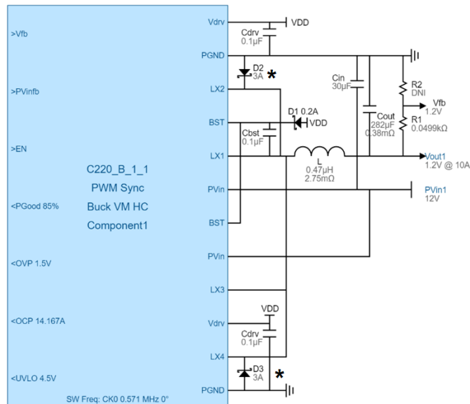
图解 1: C220_B 应用原理图
