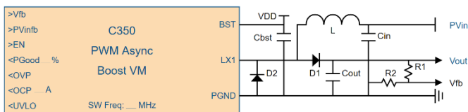
图解 1: C350 应用原理图
